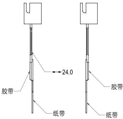
常规编带
