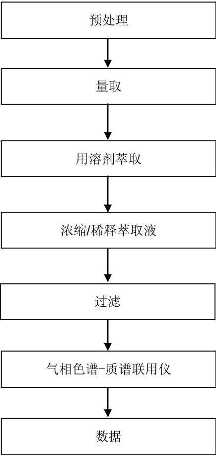
PBB/PBDE 检测流程图
