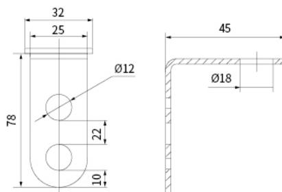
螺母侧安装式 Nut side mounting type
