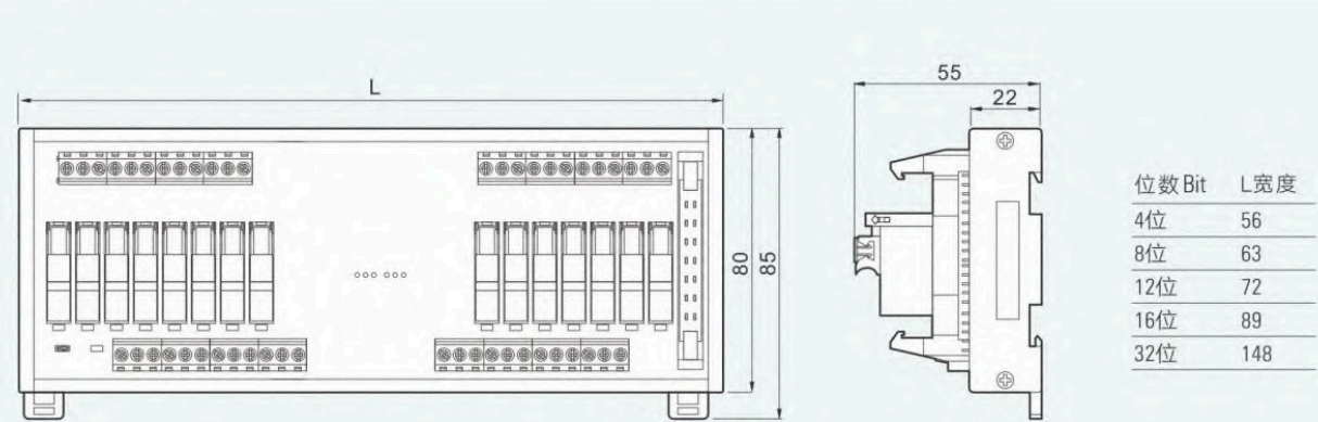
外形尺寸图 Dimensions (mm)
