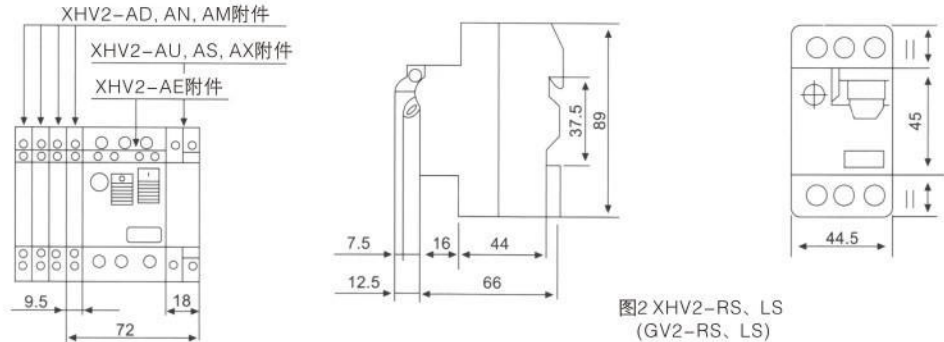
图1 XHV2-AN...,AD..., AM... XHV2-AU..., AS...,AX... XHV2-AE...
