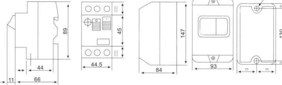
图3 XHV2-M (GV2-M)
