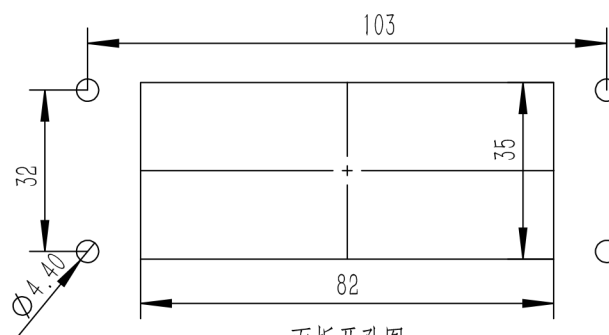
面板开孔图
