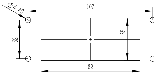
面板开孔图
