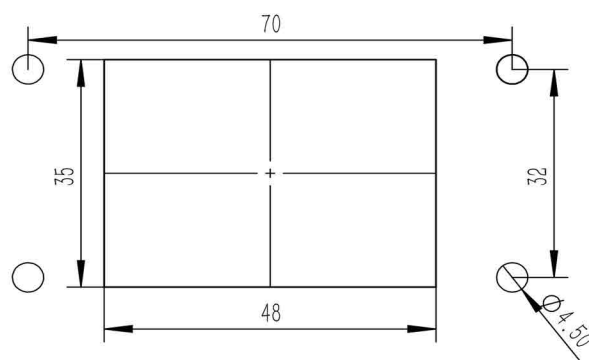
面板开孔尺寸图
