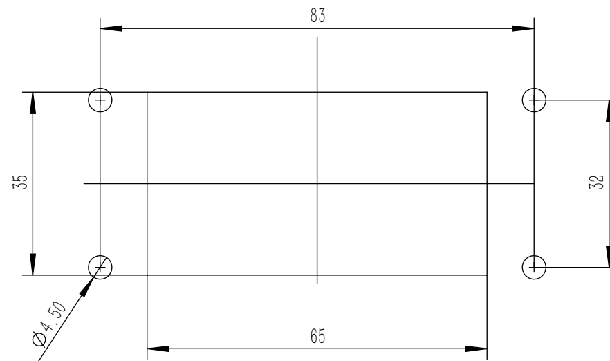
面板开孔图
