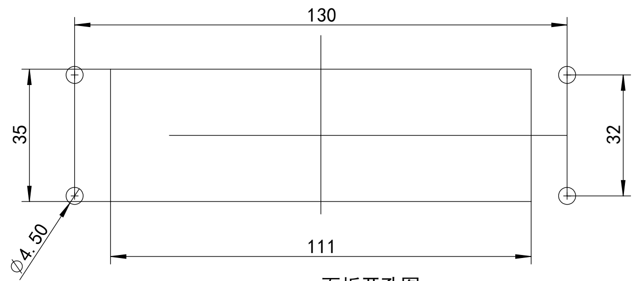
面板开孔图
