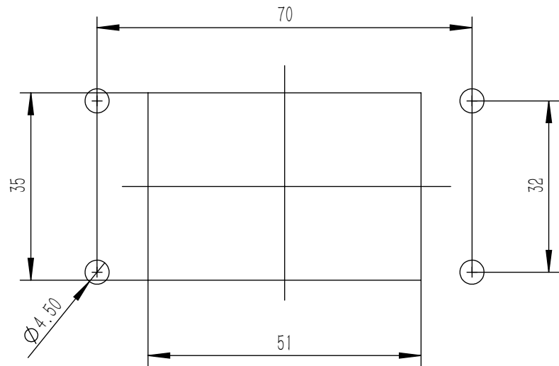
面板开孔图
