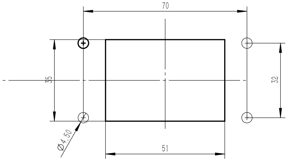
面板开孔图
