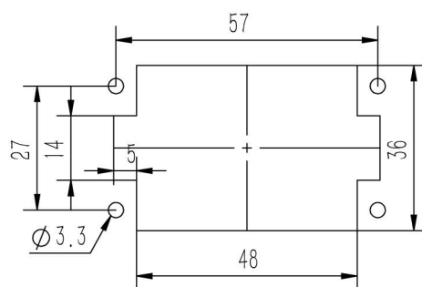
面板开孔图
