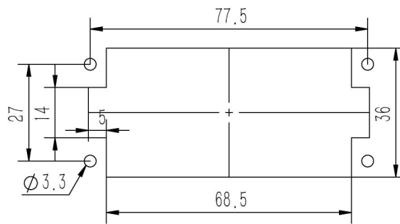
面板开孔图
