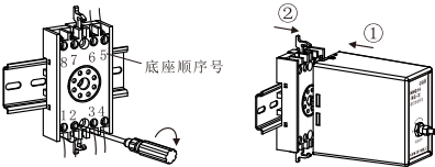
(3) 导轨式安装: 按底座顺序号接上导线并拧紧接线螺钉 (4) 导轨式安装: 装上路灯自动开关并合上挂钩
