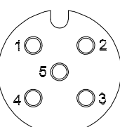
5Pin A coding
