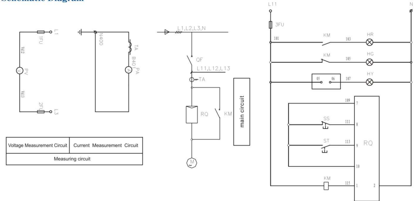
ZJRG/1T1 Wiring Diagram
