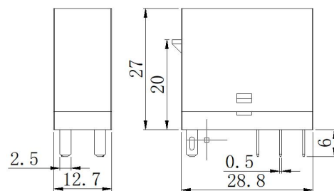
HHC69K-2Z 外形尺
