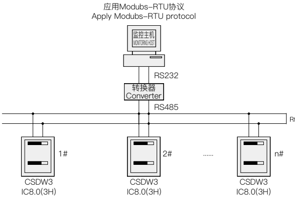
通讯组网连接示意图一 Communication Network Connection Diagram I
