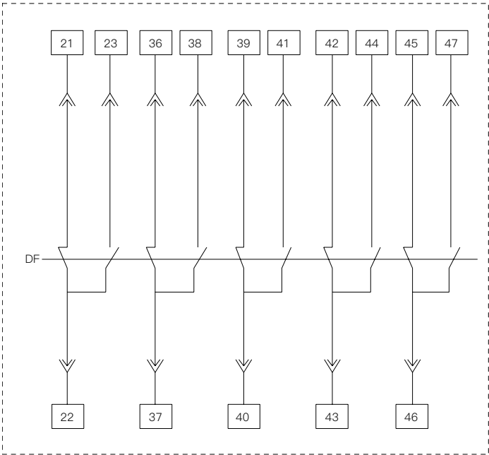
五组转换（特殊配置） Five-group conversion (special configuration)
